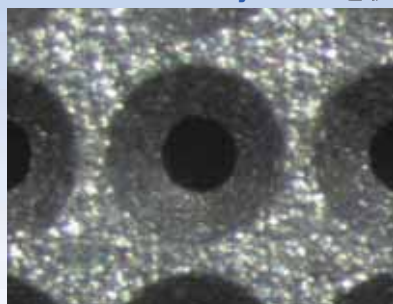
BGA 用 \phi 50 \mu\text{m} 吸着治具 ザグリ穴径の公差 1 \mu\text{m} 未満
